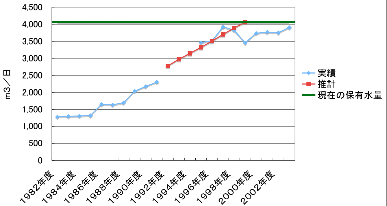
西方町上水道1日最大給水量の実績と推計
